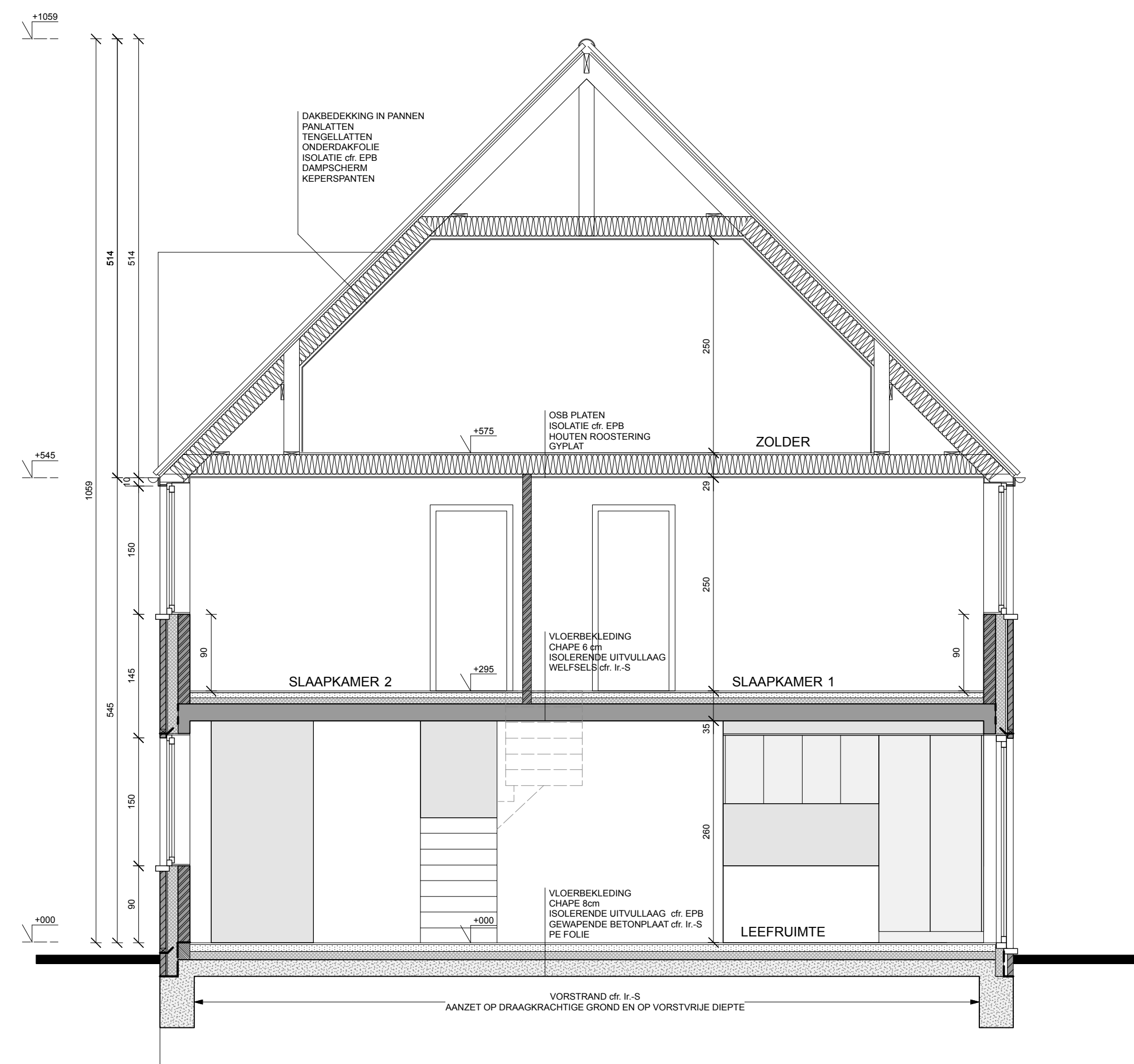
DOORSNEDE A-A SCHAAL 1/50
