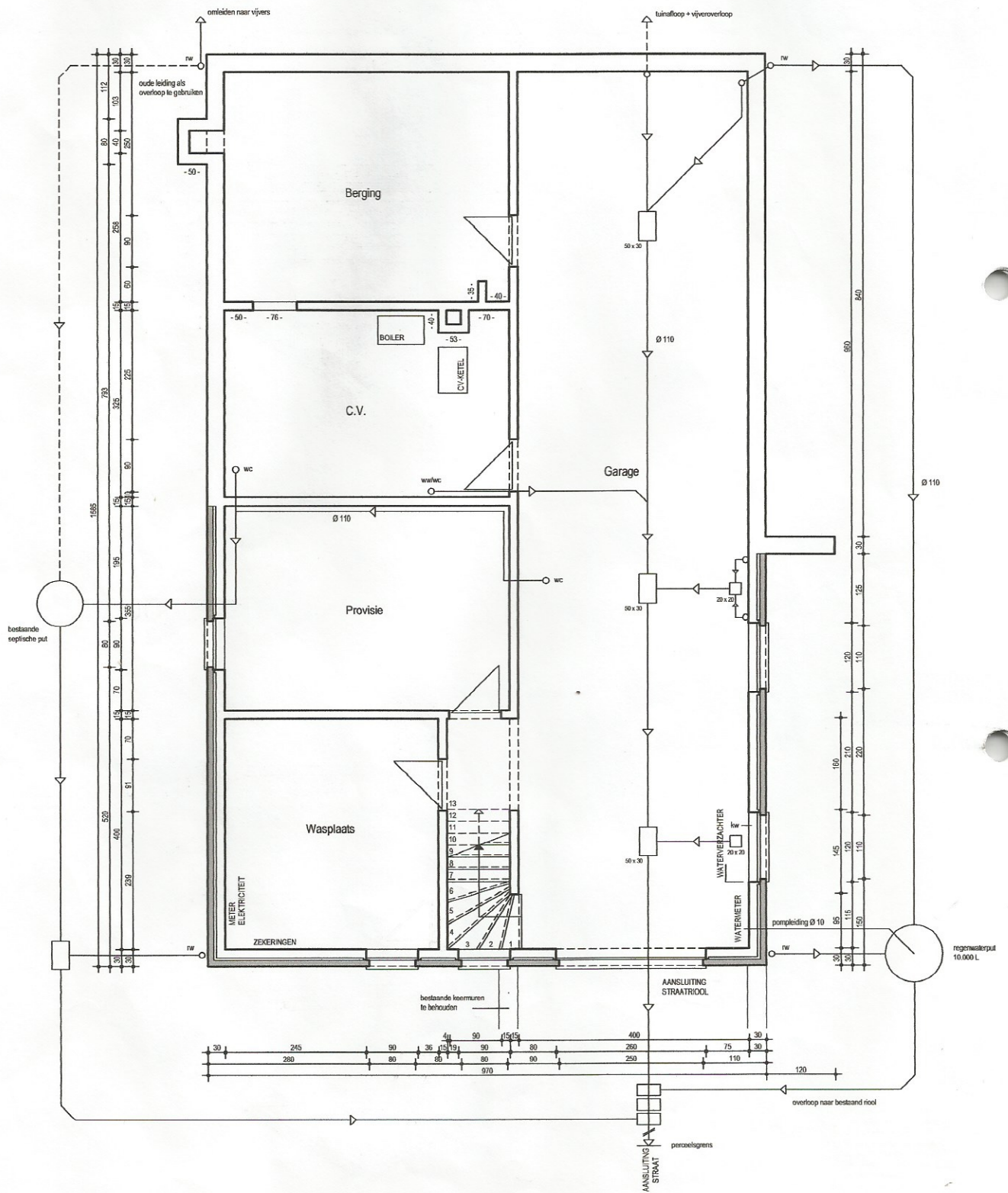
GRONDPLAN KELDERNIVEAU
